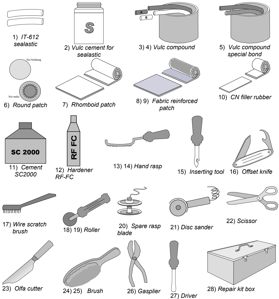
Gambar B.1 Bahan dan peralatan untuk perbaikan ringan
