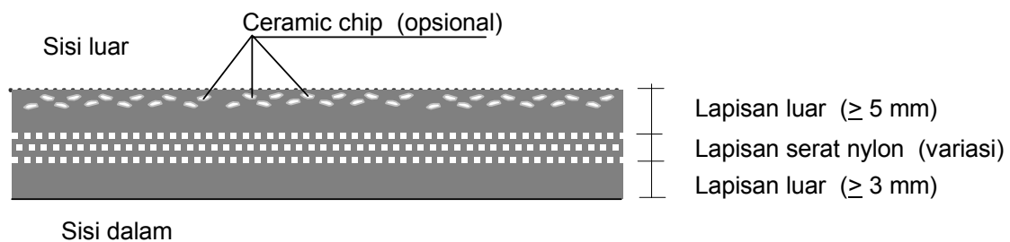
Gambar A.5 Irisan bahan karet
