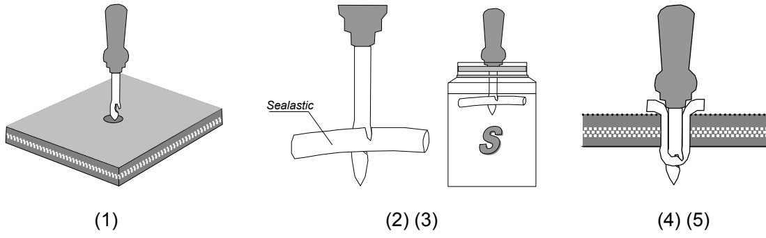
a) Penutupan lubang kecil
