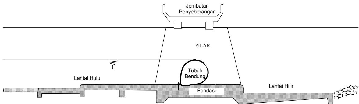
Gambar A.2 Potongan melintang tubuh bendung karet
