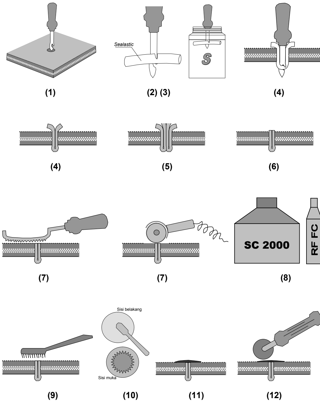
Gambar B.3 Sketsa langkah kerja perbaikan kelas A
