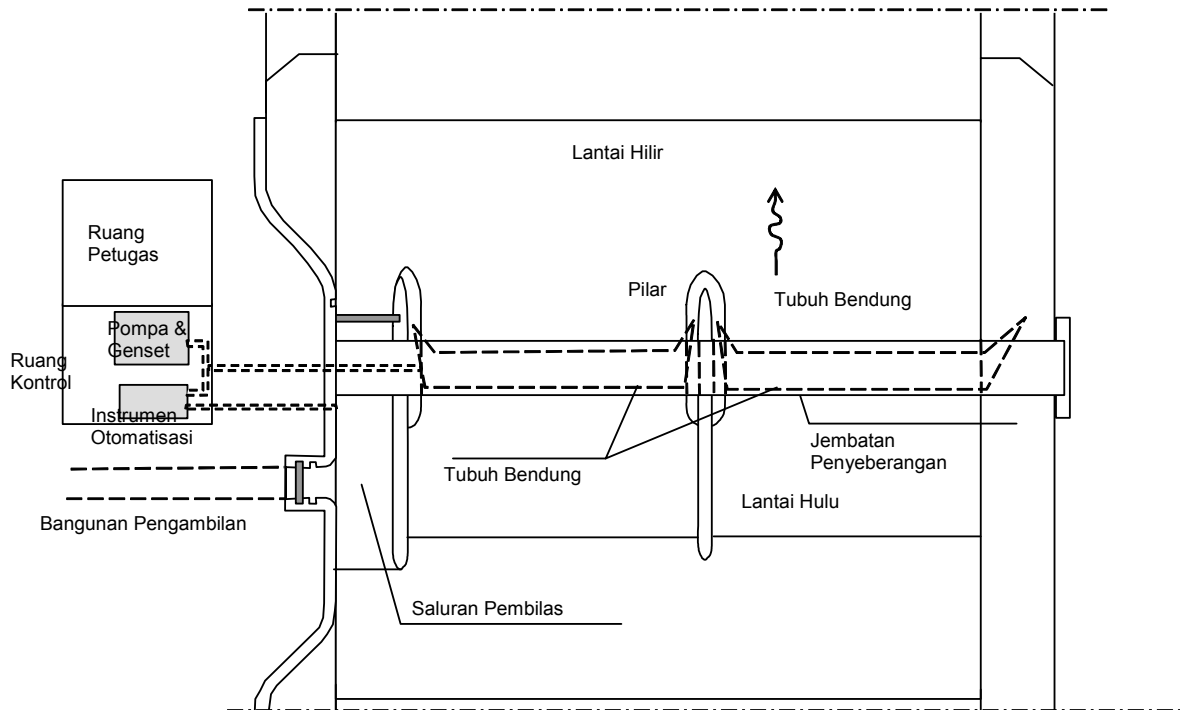
Gambar A.1 Contoh denah bendung karet
